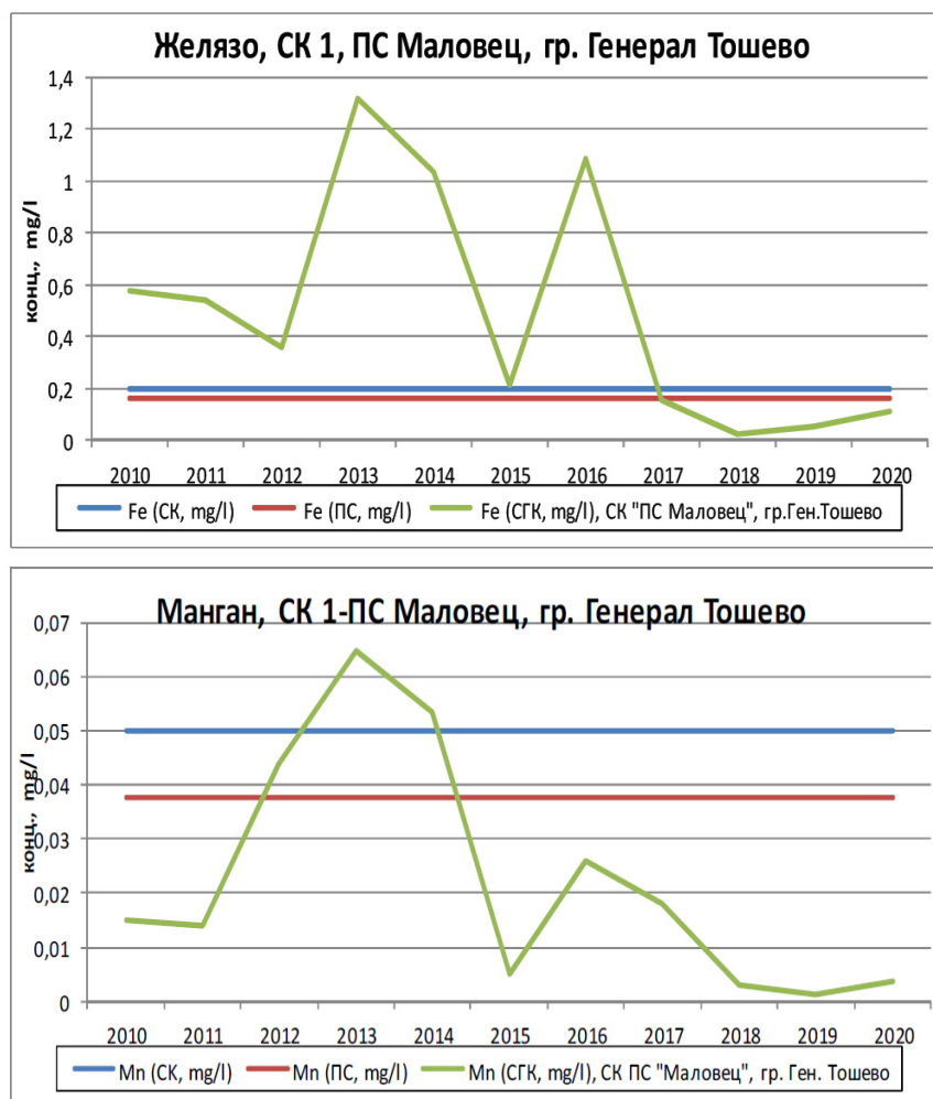
Фиг. 10: Мониторинг на водата при МП СК-ПС „Маловец“ 2010-2020 г.
