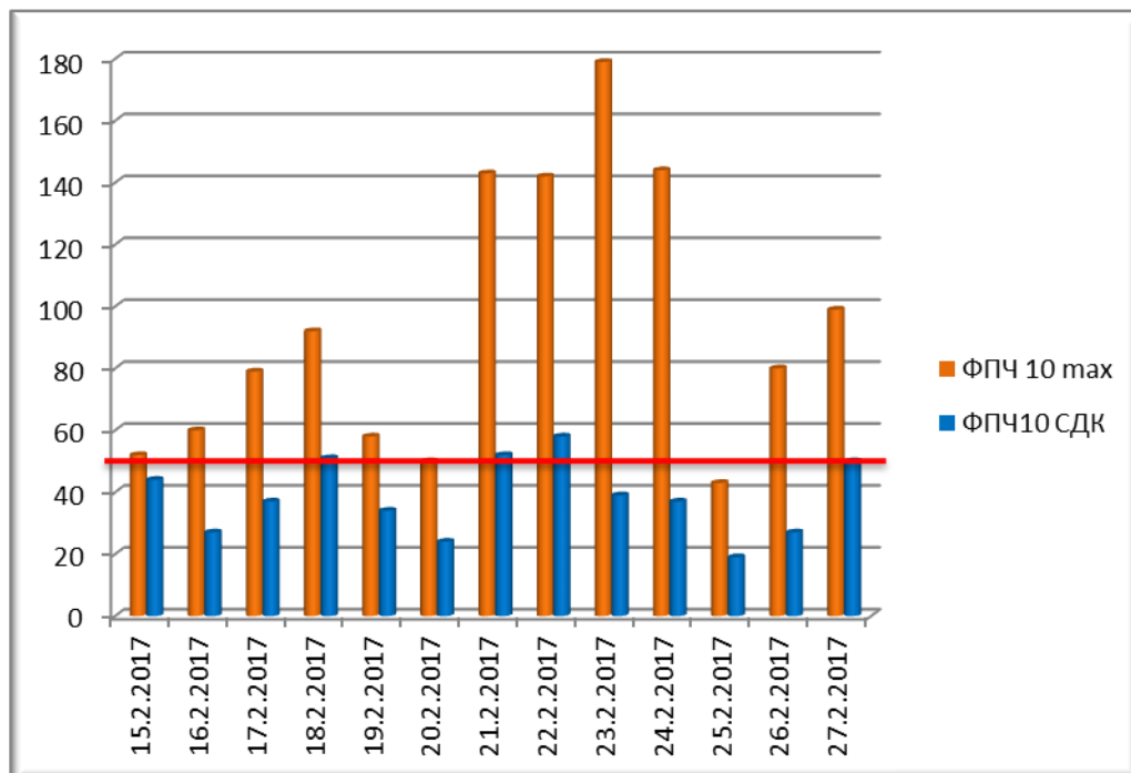
Диаграма №2 Измерени ФПЧ 10 през месец февруари 2017 г. Източник: Община Каспичан
