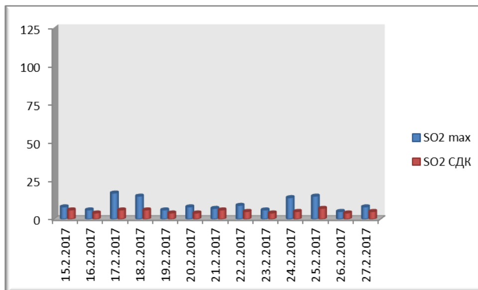
Диаграма №3 Измерен серен диоксид, Източник: Община Каспичан
