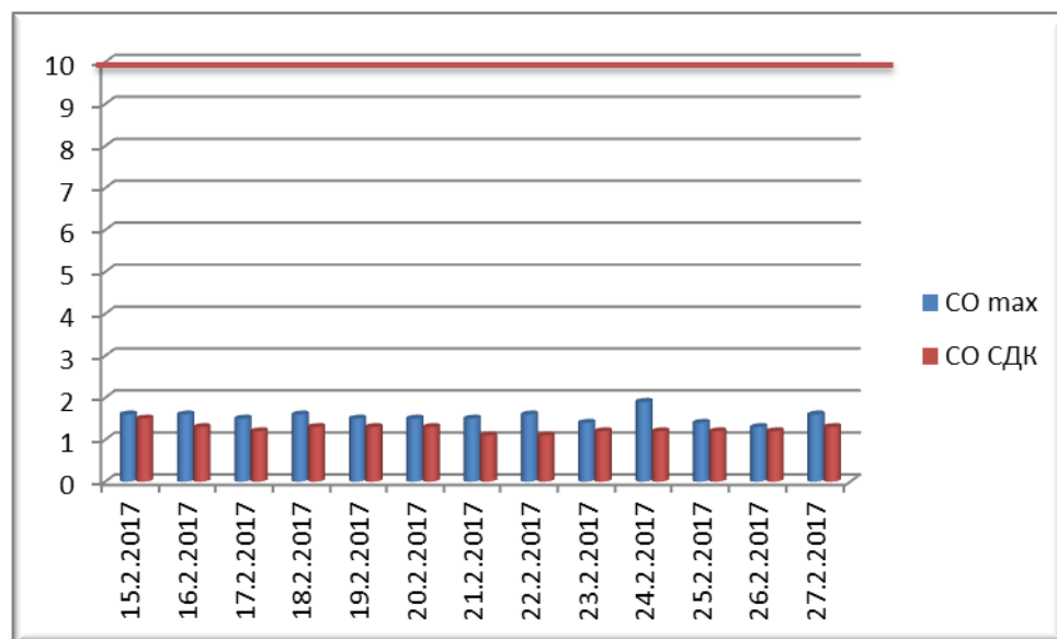
Диаграма №4 Измерени стойности на СО, февруари 2017 г.
