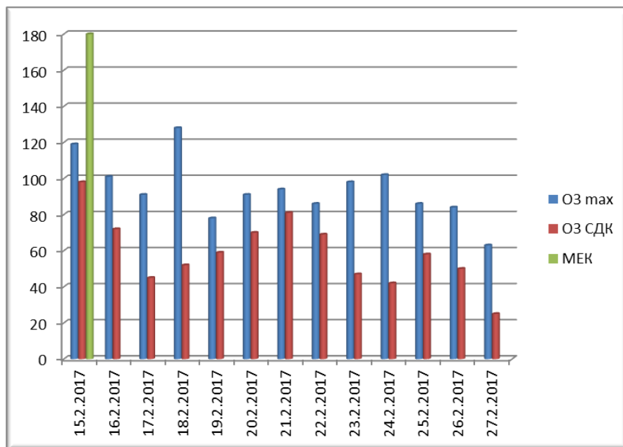
Диаграма №5 Измерени стойности на O 3 , февруари 2017 г.
