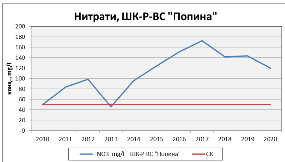
Фиг. 11: Динамиката в концентрацията на нитратни йони по години
