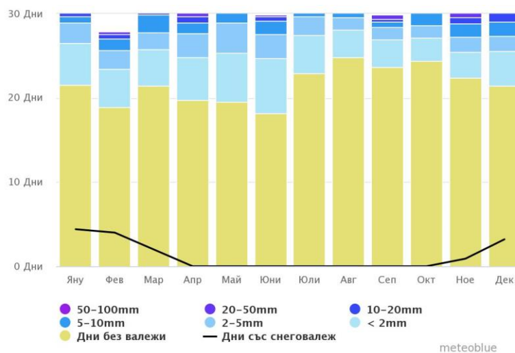
Фиг. 7: Средногодишно количество на валежите в община Ситово
