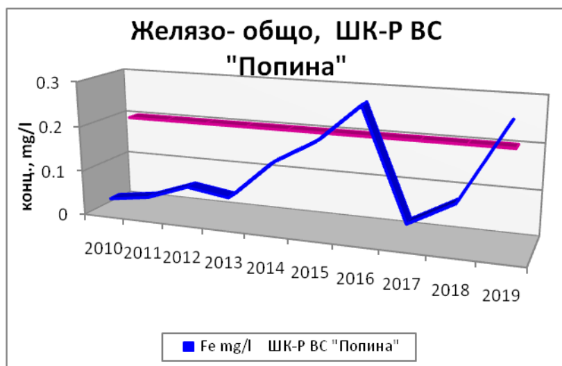
Фиг. 12: Средногодишни концентрации на показателя „желязо“
