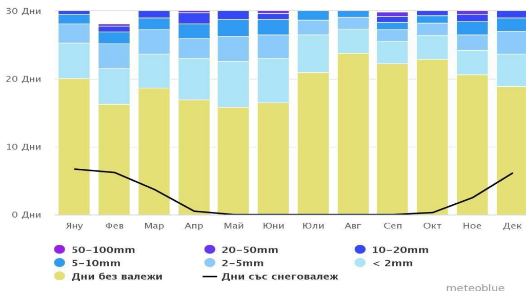
Фиг. 2: Средно количество на валежите в Елена
