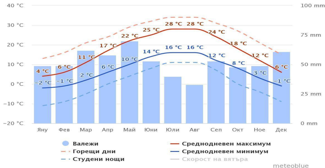
Фиг. 1: Средно месечни температури в Елена
