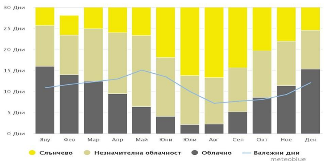
Фиг. 3: Облачни и слънчеви дни в Елена
