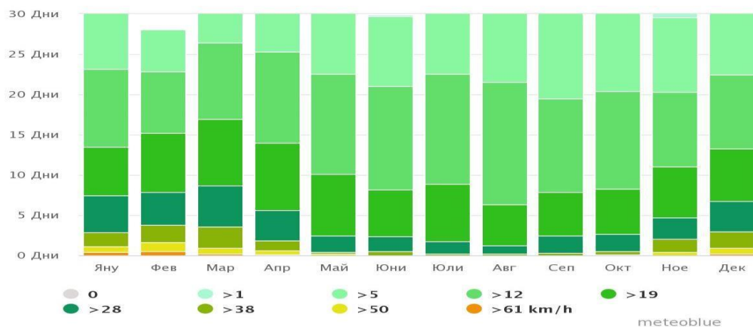
Фиг. 4: Скорост на вятъра в Елена
